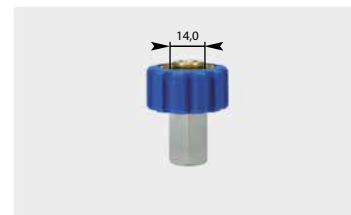
Standard 1/2" : F. Blue. Max. 400 bar / 150 °C
