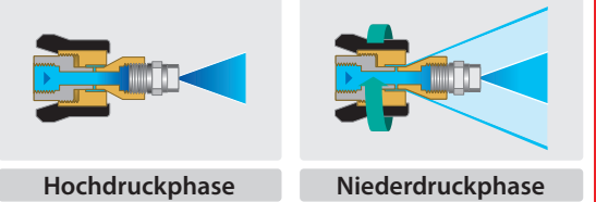
Funktionsprinzip einer Schwallregeldüse
